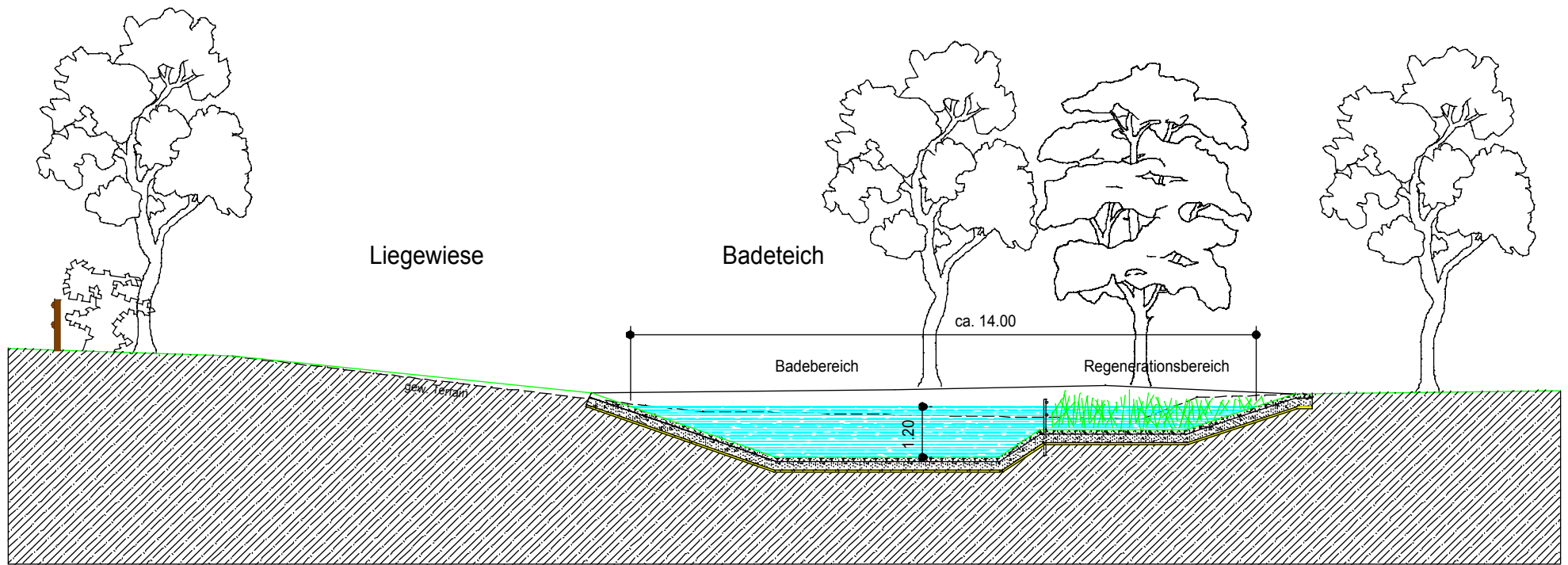
Querschnitt
